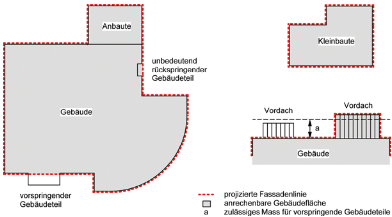
Figur 7.4 Anrechenbare Gebäudefläche
